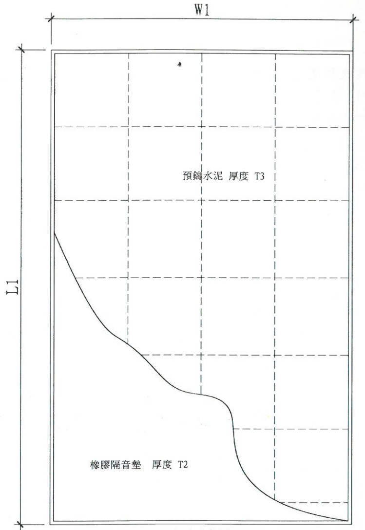
平面示意圖
