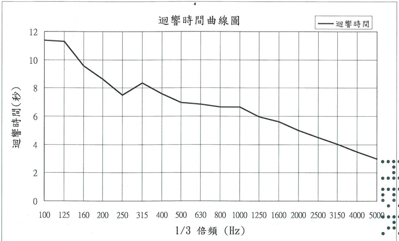
迴響時間曲線圖
